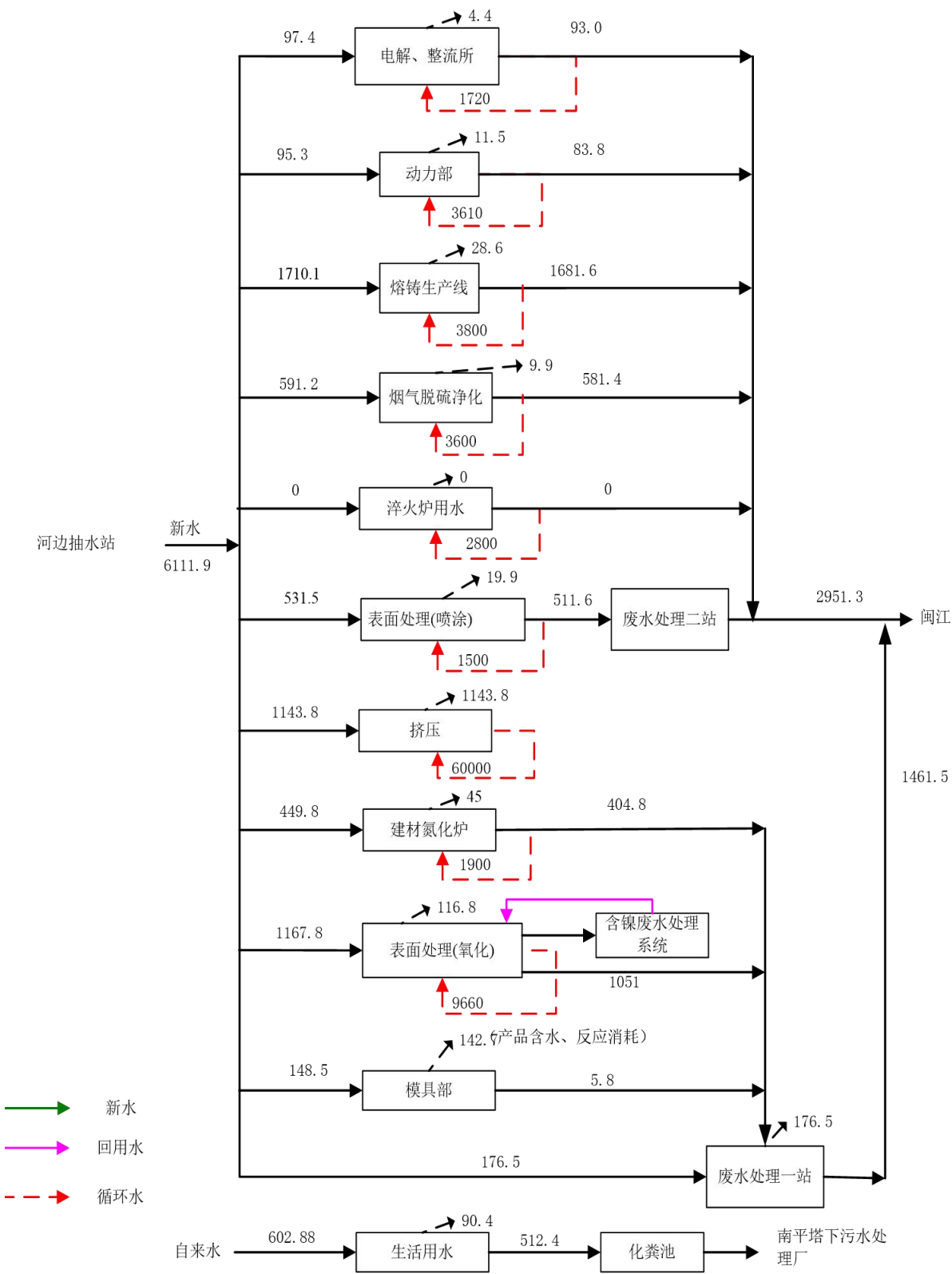
每日用水平衡图 (m 3 /d)
